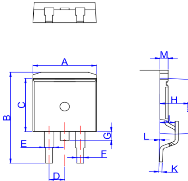
TO-263
